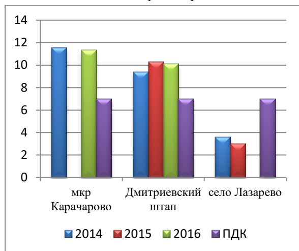
Рис. 2. Жесткость общая.
